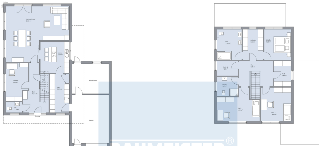
Haus Milberg Grundriss EG
