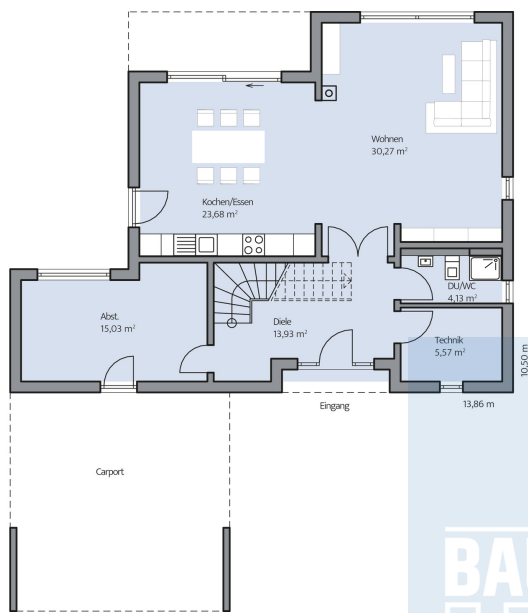
Haus Cornelius Grundriss
